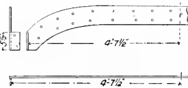
Figs. 1250-1251. End-plate Stiffener (2).
